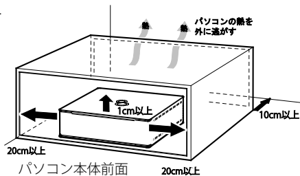
パソコン本体前面
