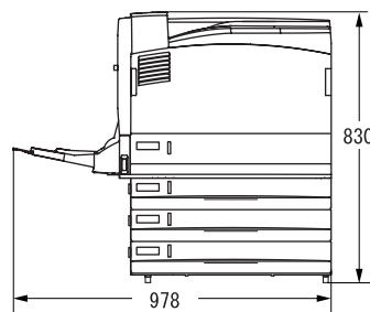
拡張給紙ユニット-B (3トレイ) 装着の場合
