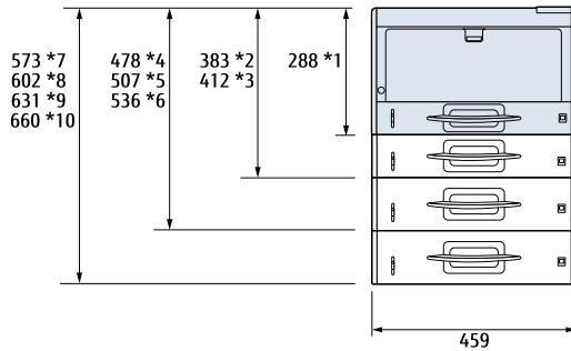
■ 正面図
