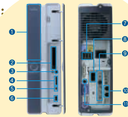
①スーパーマルチドライブ(または、DVDマルチドライブ、DVD-R/RWドライブ) ②PCカードスロット ③ヘッドホン/光デジタルオーディオ出力端子 ④SDカードメモリスティック・スロット*11 ⑤IEEE1394(DV)端子 ⑥⑦USBコネクタ ⑧モデム ⑨テレビ機能 ⑩ブロードバンドポート(LAN)*12 ⑪ビデオ出力(ビデオ)端子*13
