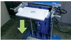
落下試験
