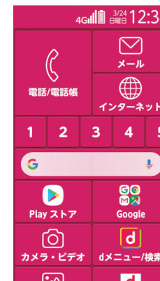
(ホーム画面)
