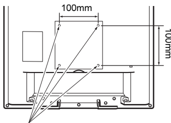
アーム、壁掛けキット固定用ネジ穴
