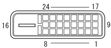
端子配列図
