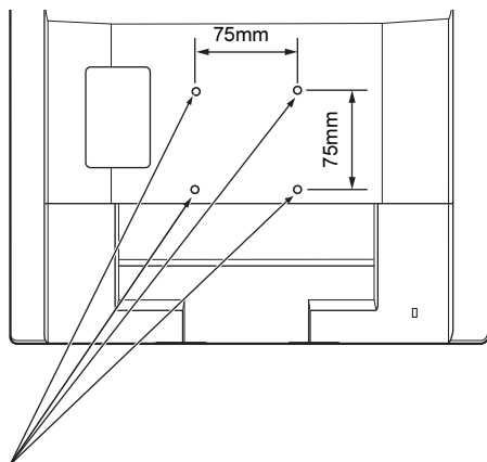
アーム、壁掛けキット固定用ネジ穴
