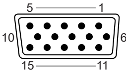
端子配列図
