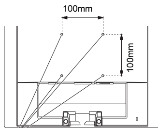
アーム、壁掛けキット固定用ネジ穴
