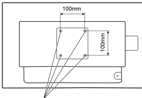
アーム、壁掛けキット固定用ネジ穴
