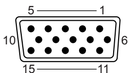
端子配列図
