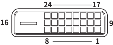
端子配列図
