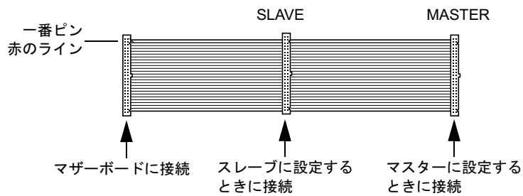
<セカンダリ IDE 用ケーブル (40 芯)>
