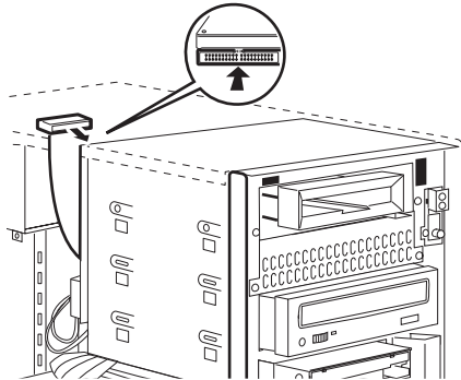
<セカンダリ IDE 用ケーブル (40 芯)>
