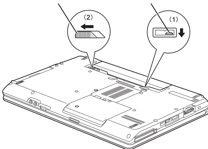
内蔵バッテリーパックロック2
