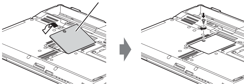
メモリスロットカバー
