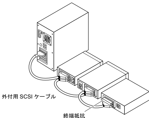
図 2. 外付用 SCSI デバイスのデージーチェーン接続
