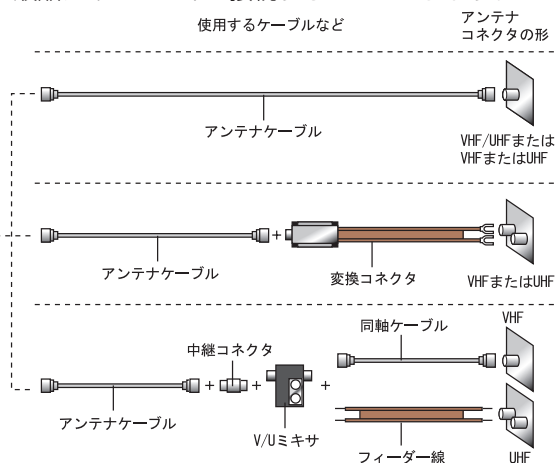
アンテナ入力 (F型同軸) 端子
