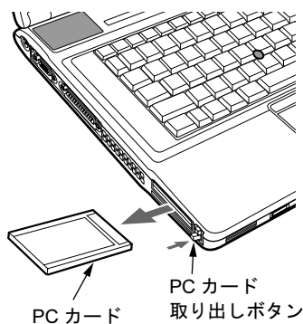
PC カード
