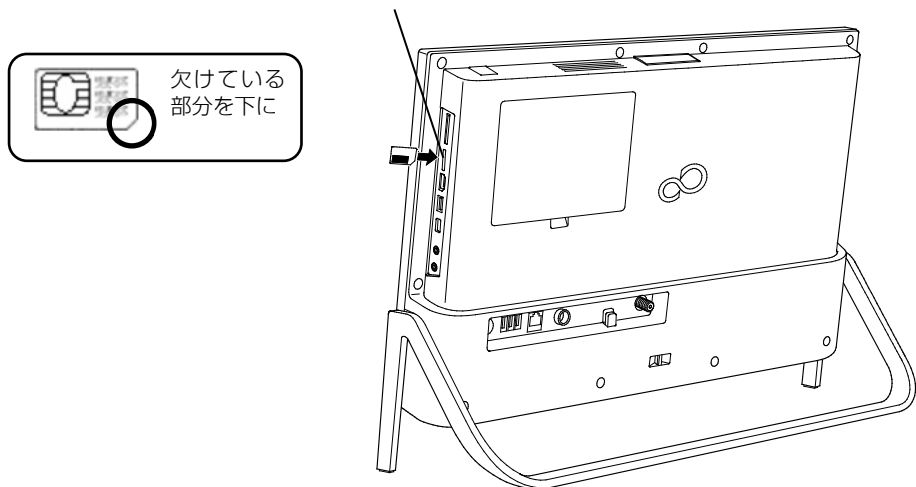
miniB-CAS カードスロット
