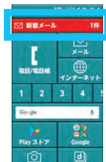
(ホーム画面)
