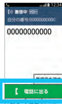
(着信画面)
